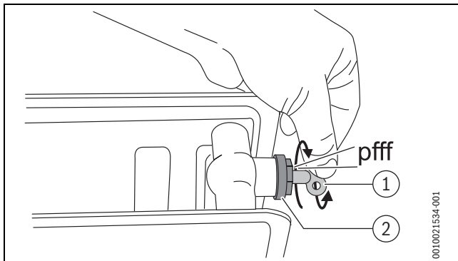
Rys. 13 Odpowietrzanie grzejników
