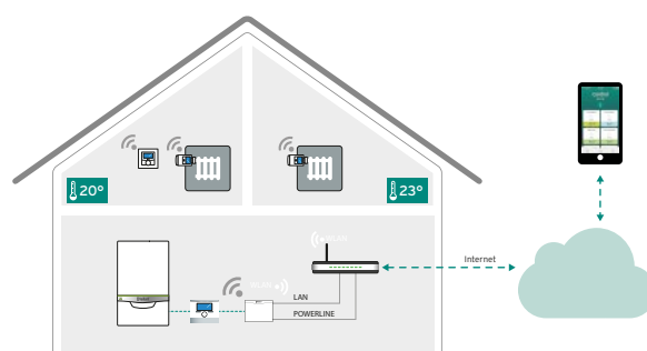
Schemat działania systemu regulacji temperatury ambiSENSE
